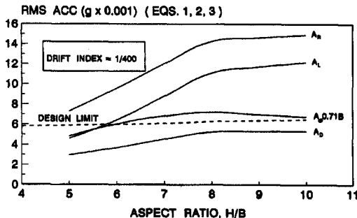
Fig. 9. Parametric study—150-ft sq bldg.
